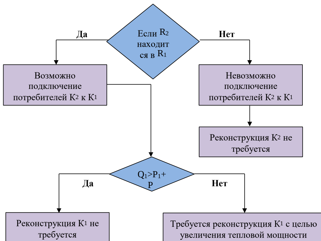
Рисунок 2.1.3 – Блок-схема обоснования реконструкции котельной K_1 , K_2 – Котельные №1 и №2;
